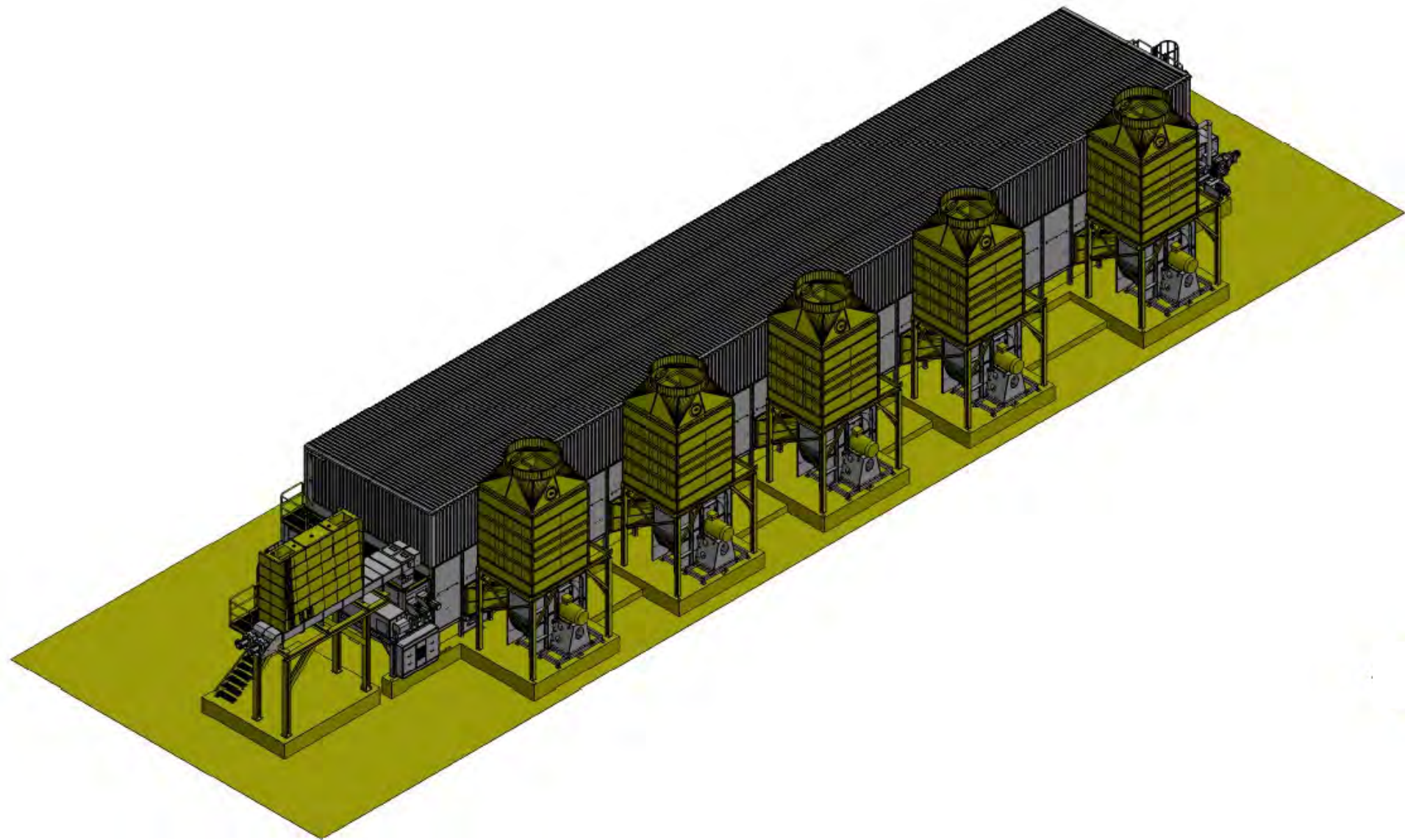
项目地：太阳纸业，广西 | 型号：BT 1/6200-39 | 预计安装年份：2025 干燥物料：桉树片 | 出料能力：约10.4 吨/小时 | 降水区间：55% - 5%湿度
