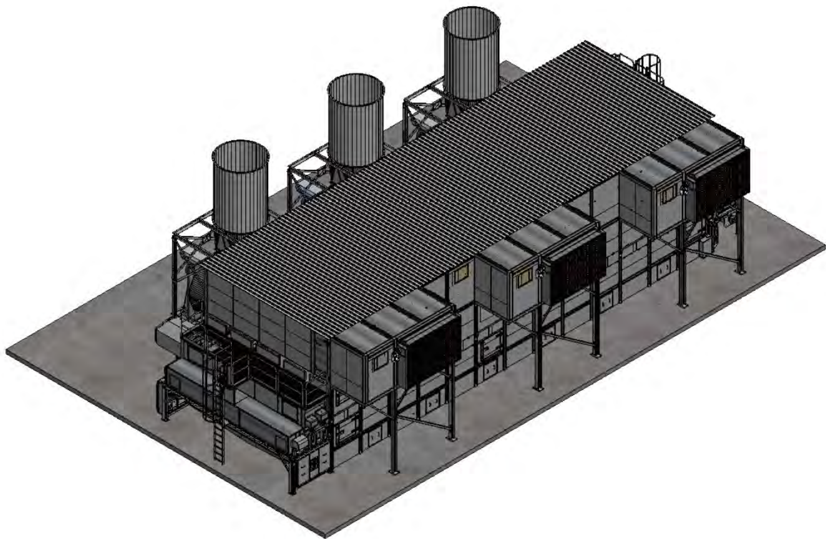
项目地：东加红狮水泥，印尼 | 型号：BT 1/6200-19.5 | 预计安装年份：2025 干燥物料：褐煤 | 出料能力：约24.7 吨/小时 | 降水区间：30% - 15%湿度
